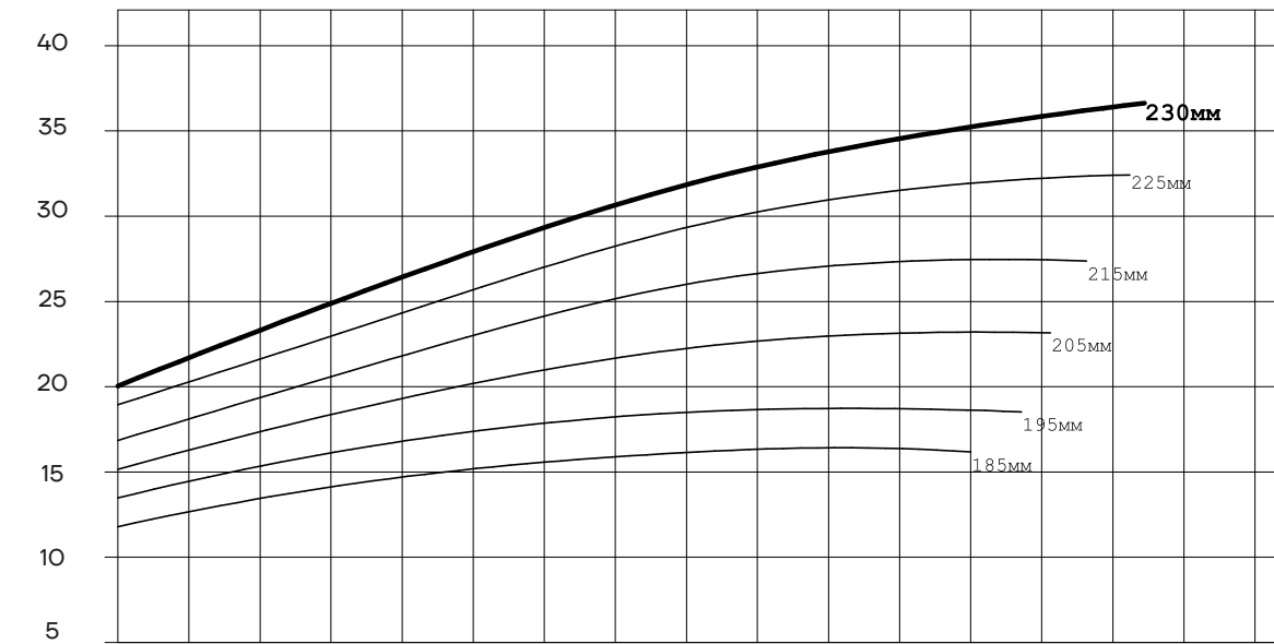
Р [кВт] на валу насоса
